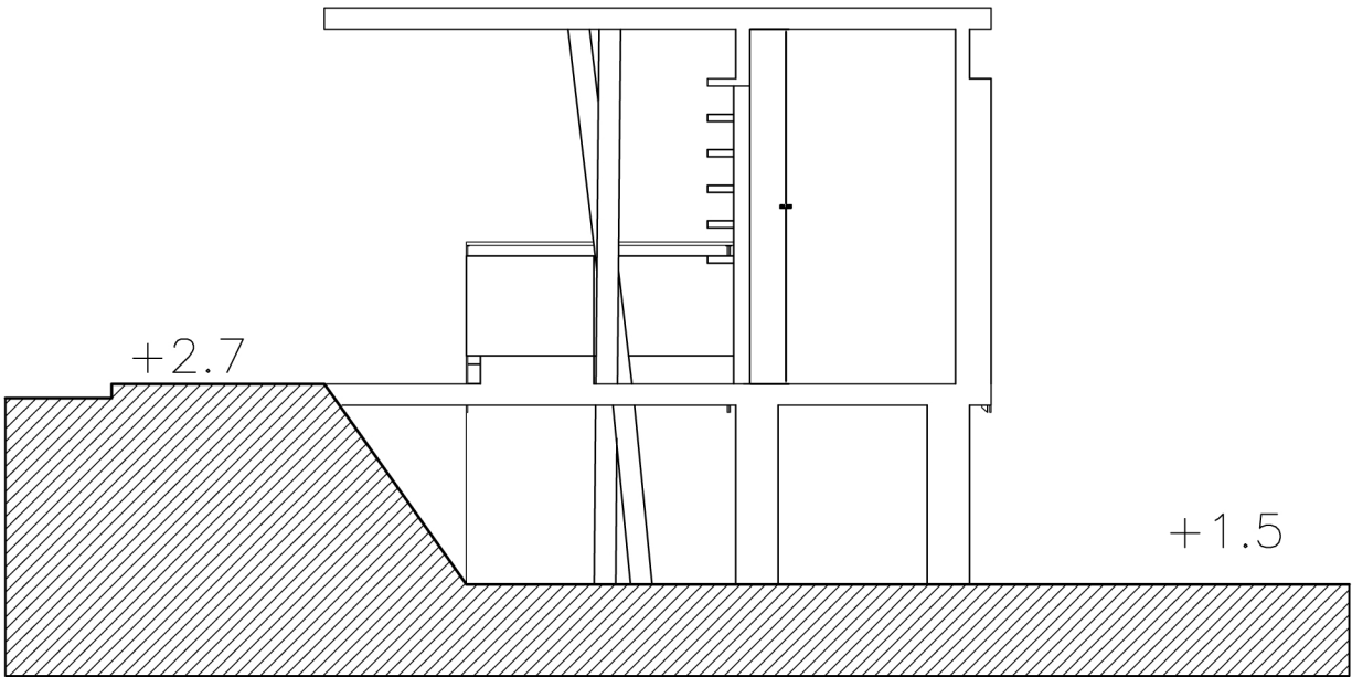
Sezione
