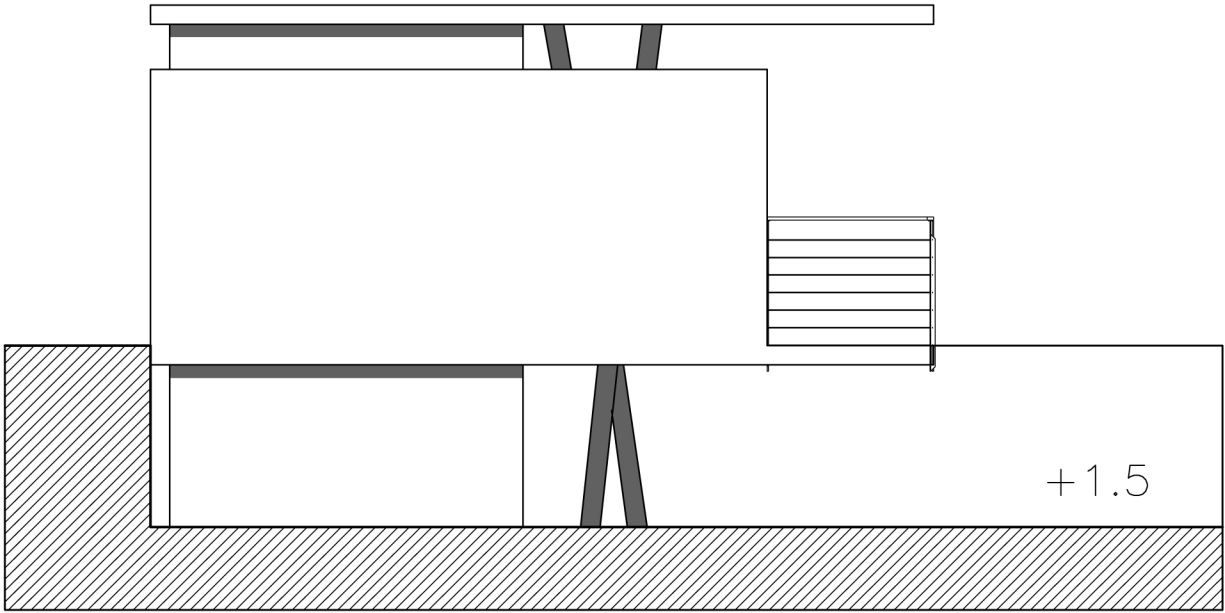
Prospetto lato spiaggia
