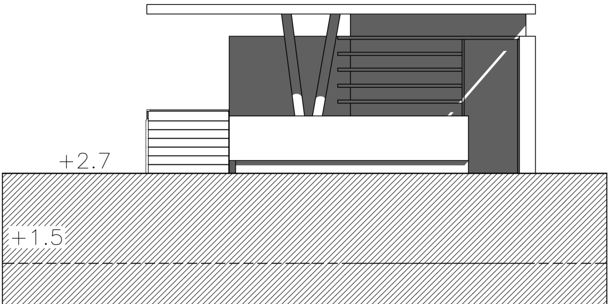
Prospetto principale
